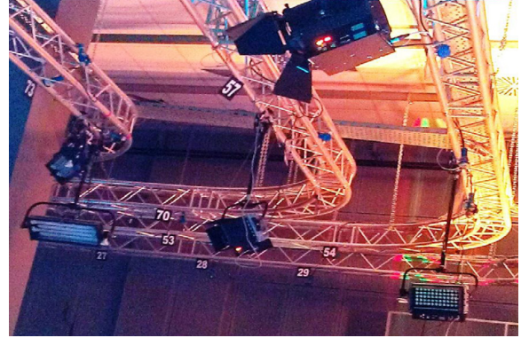
Arim-557 Led'li Spot Projektör ve Soğuk Işıklar (TRT Spor Arim- Haber Stüdyosu)
